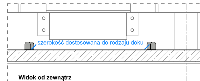
Widok od zewnątrz
