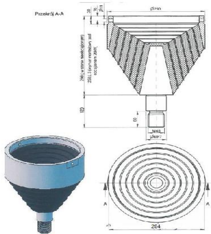
Nazwa części Sprężyna gumowo-metalowa (stożkowa) RL-4785-1 Ciężar 940 31,0
