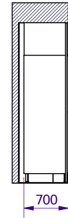
A-A ( 1 : 60 )
