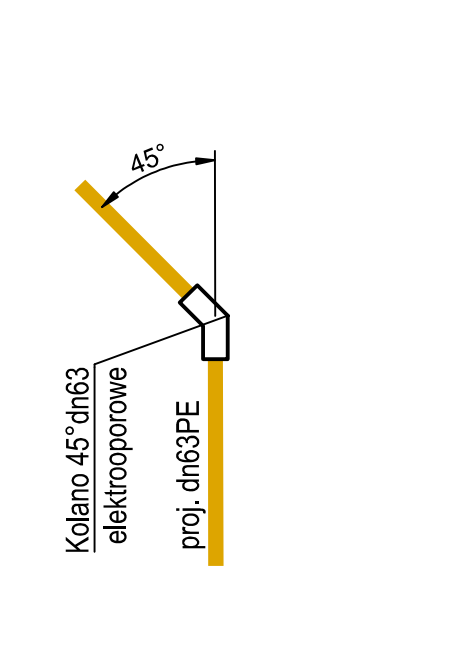
SCHEMAT WĘZŁA "G11"
