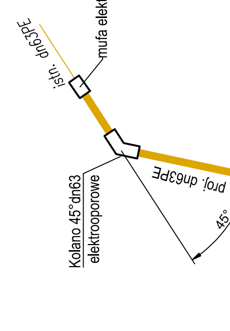
SCHEMAT WĘZŁA "D"
