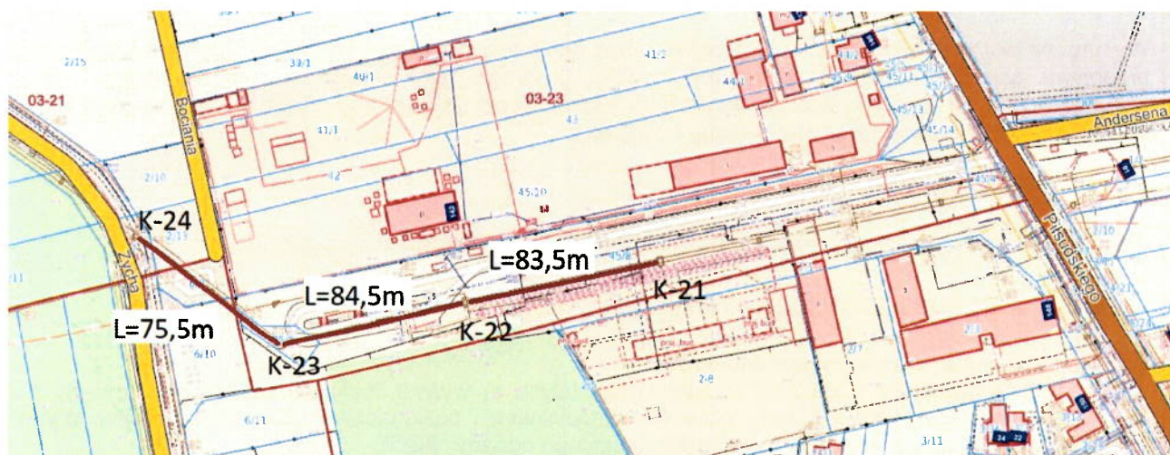
Rys.1 Kolektor ściekowy w ul. Sezatkowej w Żąbkach i Klamrowej w Warszawie.
