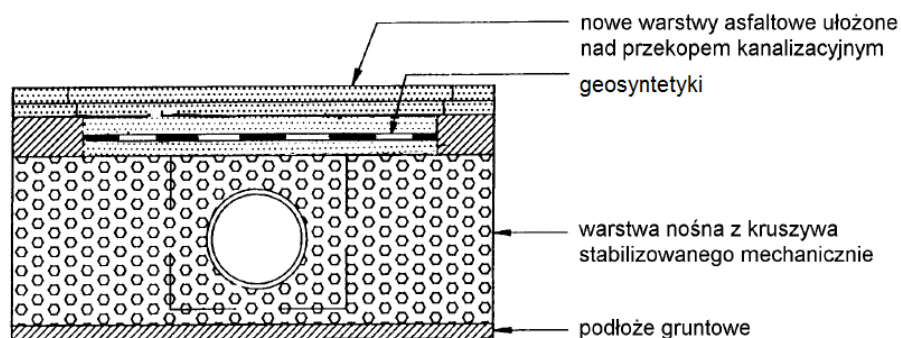
Rys. 6. Wzmocnienie nawierzchni pod przekopem kanalizacyjnym
