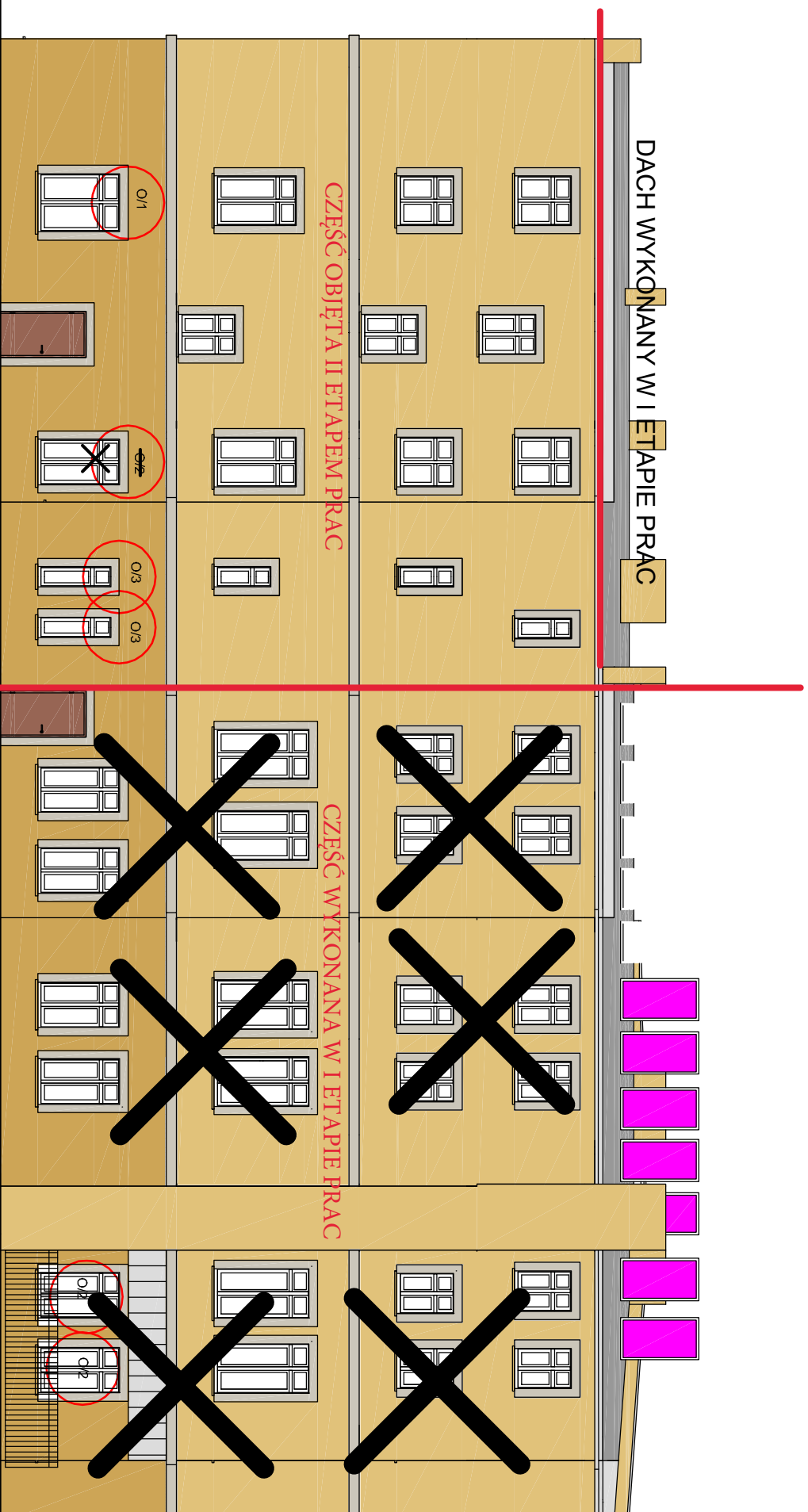
elewacja południowa
