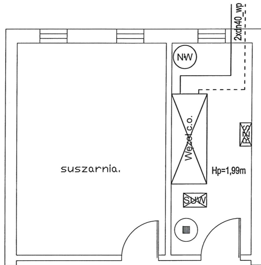
STAN ISTNIEJĄCY
