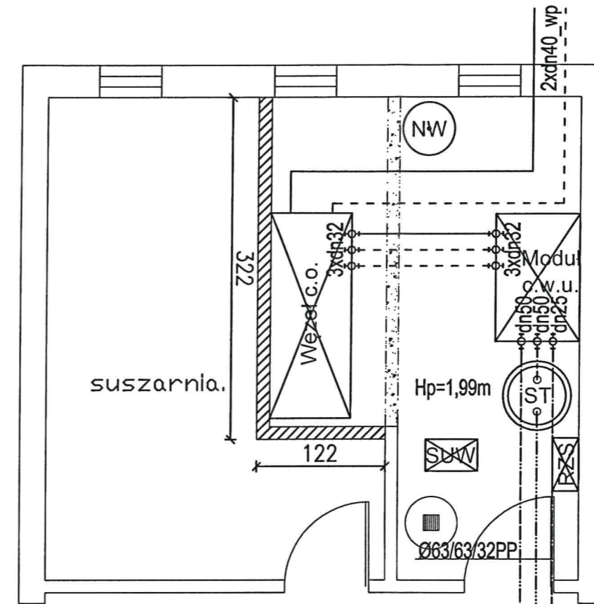
STAN PROJEKTOWANY
