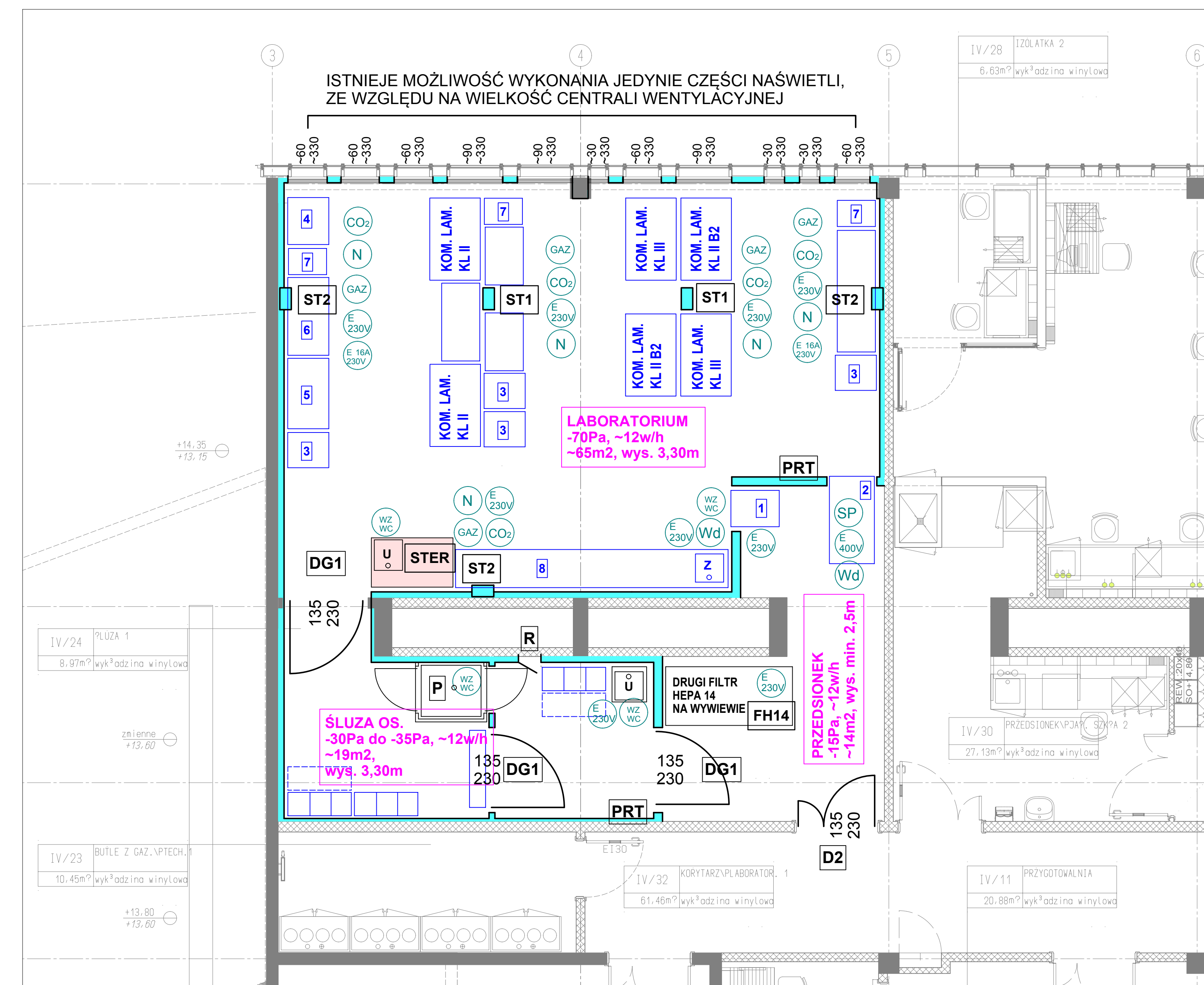
RZUT LABORATORIUM BSL3+ - ZAŁOŻENIA IV KONDYGNACJA NADZIEMNA SKALA 1:50
