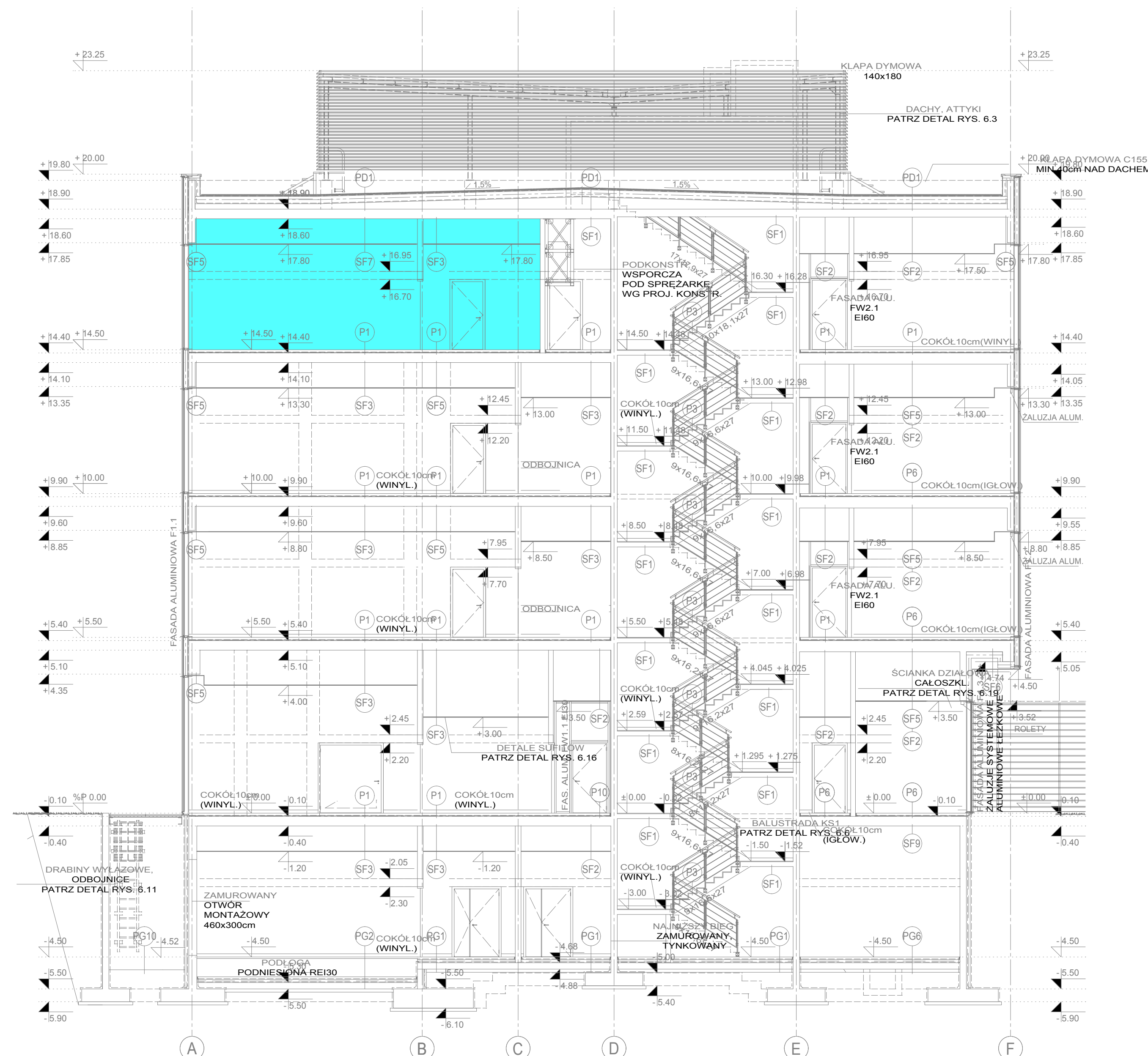
USYTUOWANIE LABORATORIUM BSL3+ IV KONDYGNACJA NADZIEMNA SKALA 1:100
