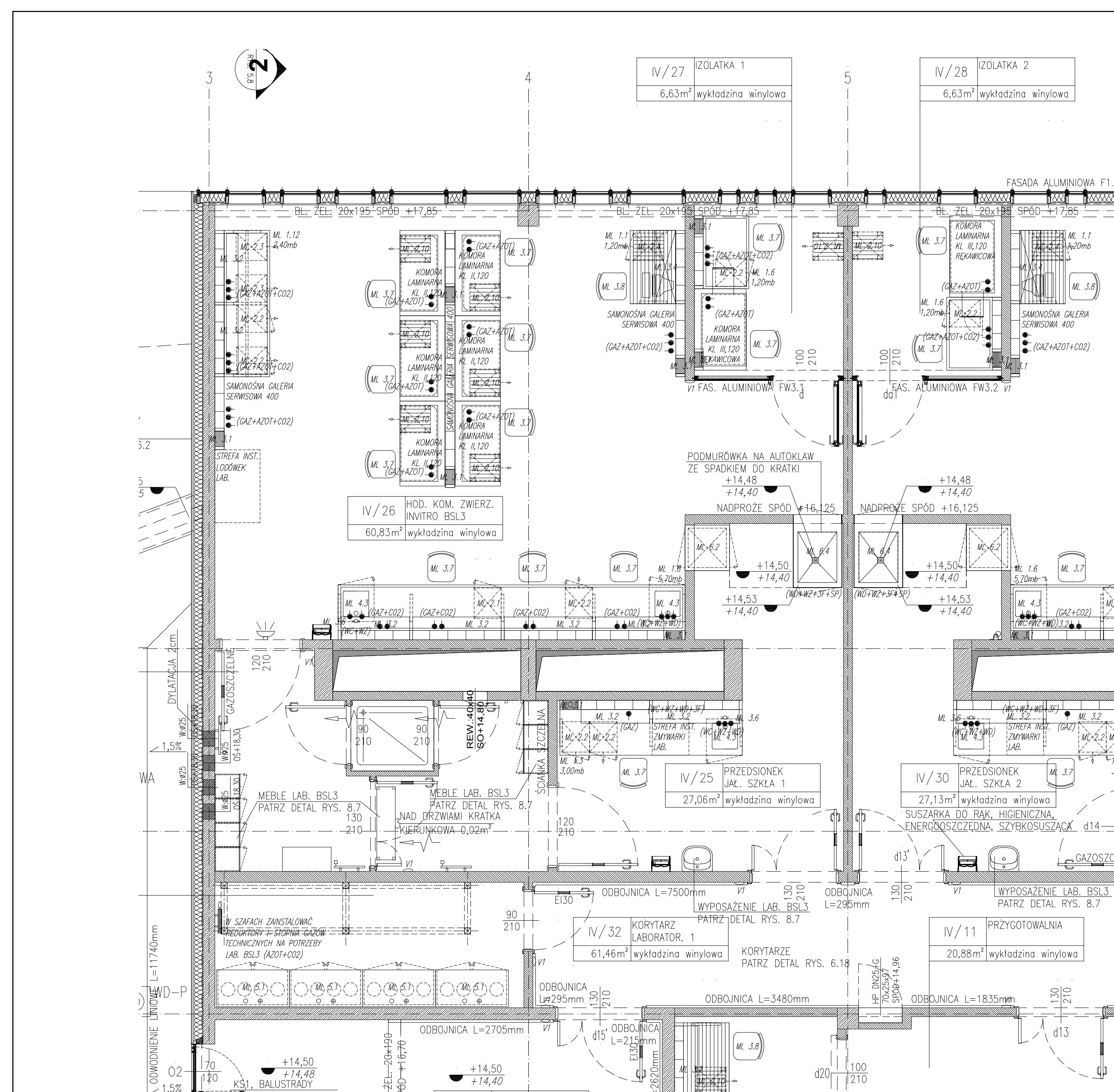
RZUT ISTNIEJĄCEGO LABORATORIUM IV KONDYGNACJA NADZIEMNA SKALA 1:50
