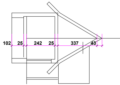
PRZEKRÓJ
