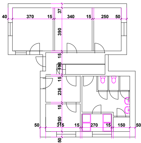
RZUT PARTERU
