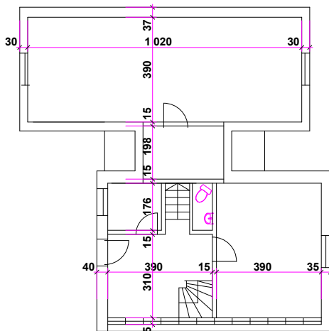
RZUT PIĘTRA
