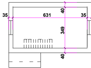
RZUT PIĘTRA
