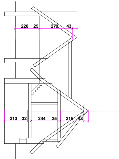
PRZEKRÓJ
