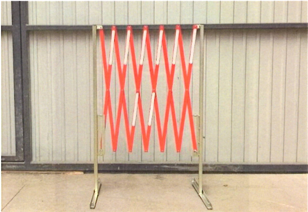
Rys. 3. Stalowa zapora nożycowa rozsuwana z płaską podstawą
