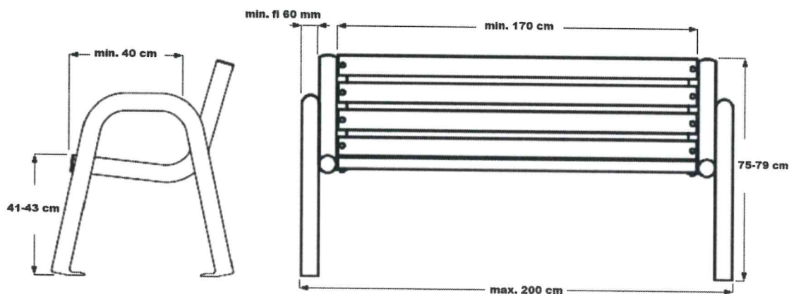
Rys. Wymiary ławki
