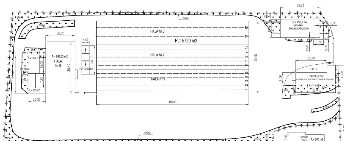
PLAN SYTUACYJNY OBIEKTÓW NA TERENIE ZAJEZDNI TRAMWAJOWEJ NR 1 ul. Kamienna 74
