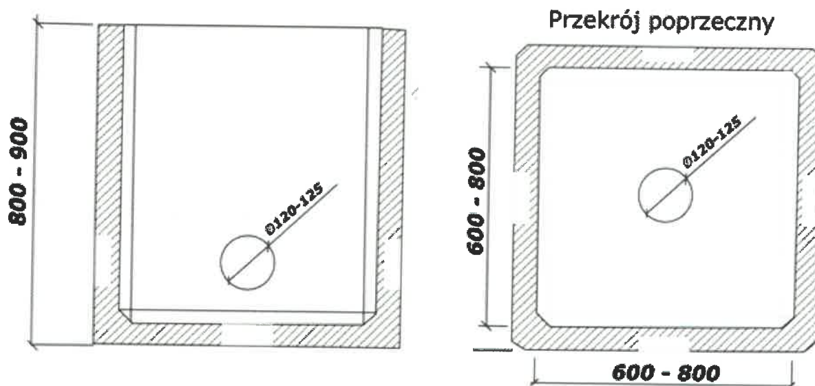
Rys. Studnia kablowa.
