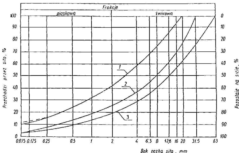
rys. nr 1 pole dobrego uziarnienia kruszyw przeznaczonych na podbudowy wykonywane metodą stabilizacji mechanicznej (1-2 kruszywo na podbudowę zasadniczą 1-3 dotyczy podbudowy pomocniczej)
