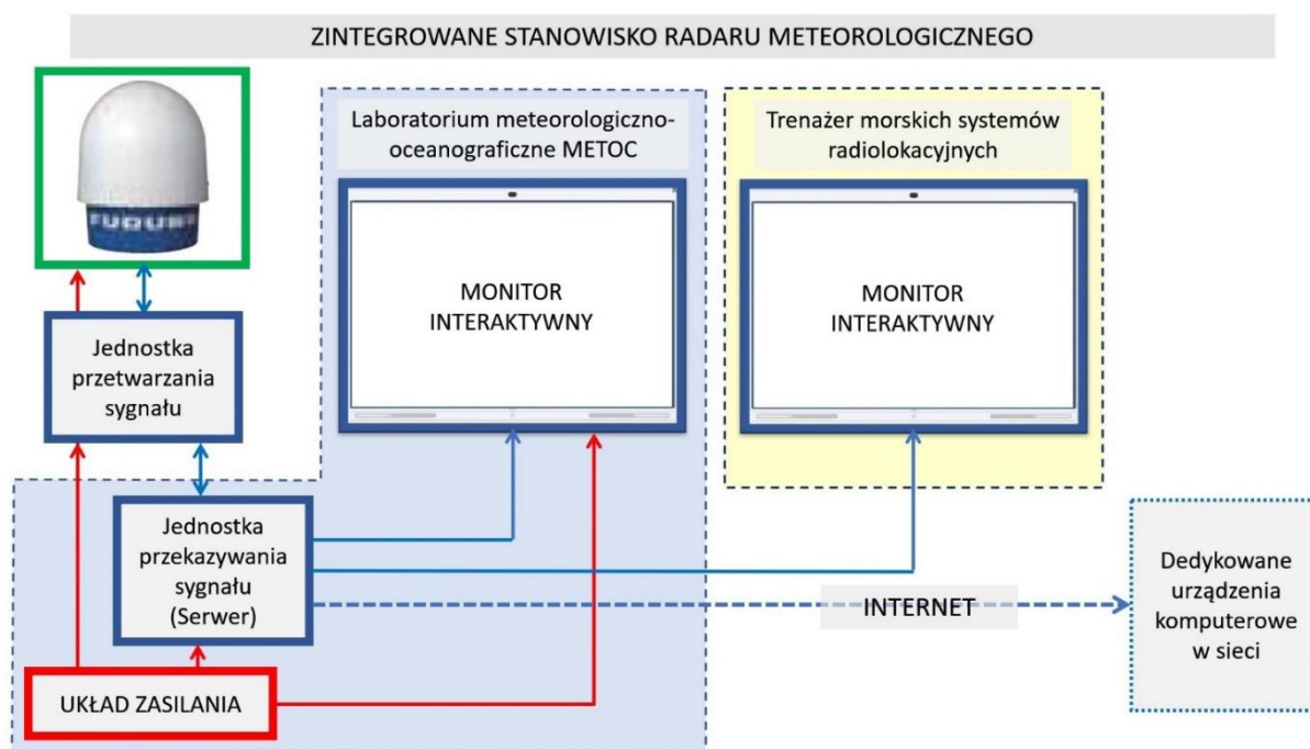
Rys. 1. Ogólne zobrazowanie zintegrowanego stanowiska radaru meteorologicznego
