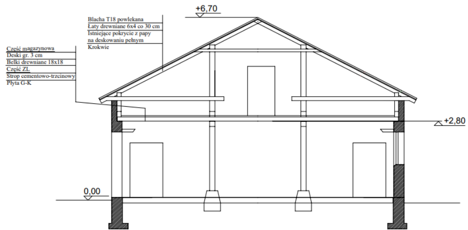
Rys. Przekrój budynku administracyjno - socjalno - magazynowego
