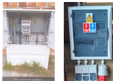
b) Budynek nr 1 – złącze kablowe, rozdzielnia główna
