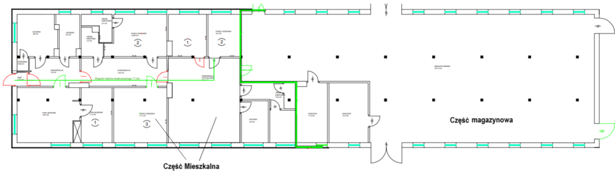
Rys. Schemat kondygnacji budynku administracyjno - socjalno - magazynowego
