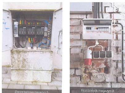
f) Budynek nr 3 – złącze kablowe, rozdzielnia główna
