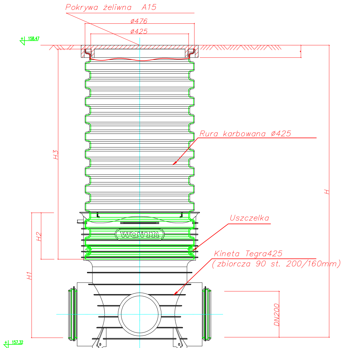
Studzienka inspekcyjna Tegra 425 z pokrywą żeliwną klasy A15
