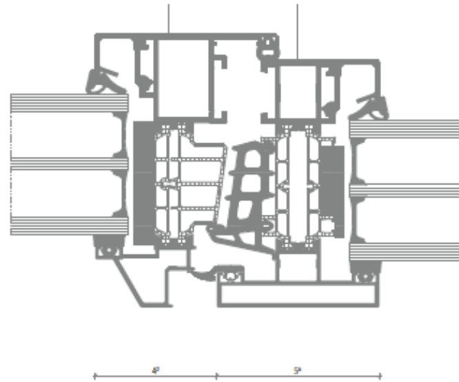
PRZEKRÓJ POZIOMY PROFLE ALUMINIOWE ALUPROF MB FERROLINE Profil INDUSTRIAL RAL 9006
