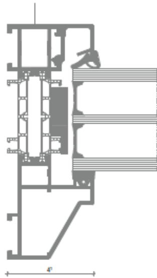
PRZEKRÓJ POZIOMY PROFLE ALUMINIOWE ALUPROF MB FERROLINE Profil INDUSTRIAL RAL 9006
