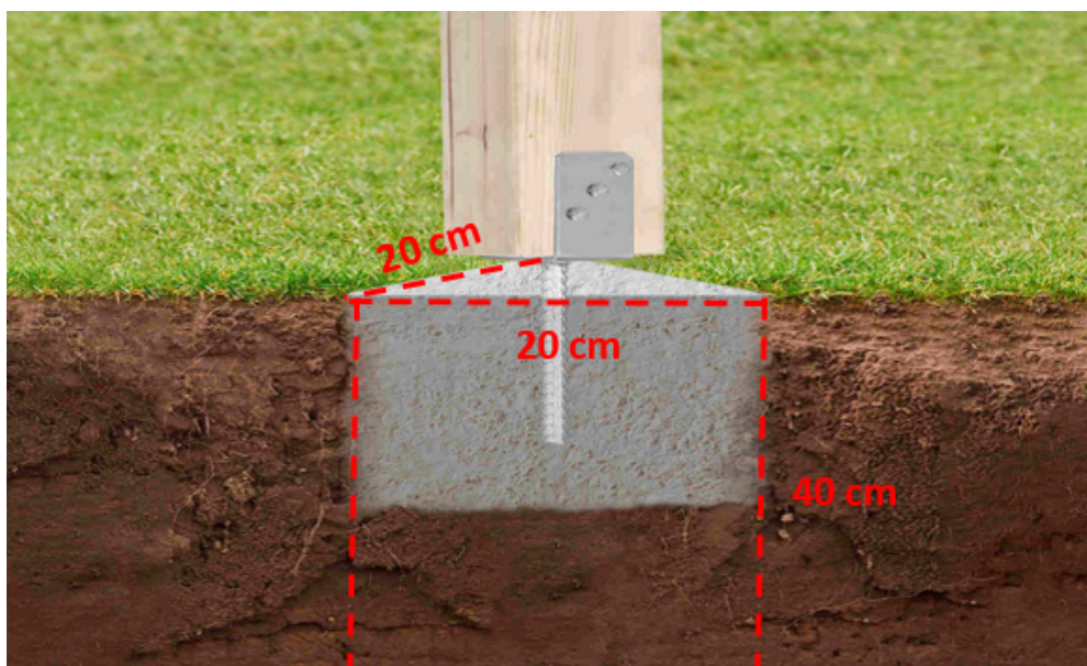
Ryc. 3 Sposób montażu
