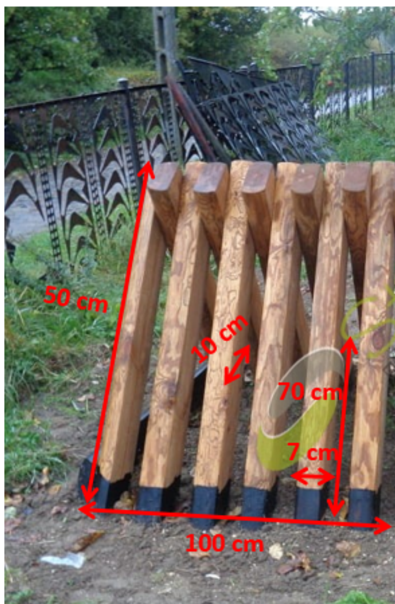
Ryc. 4. Wzór stojaka z wymiarami
