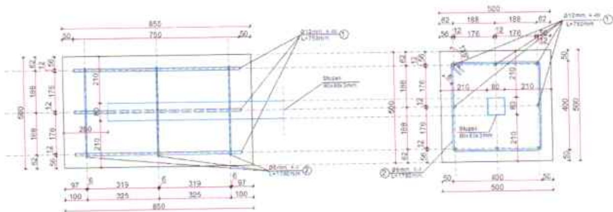
Rys. 3 Przekrój przez fundament żelbetowy.
