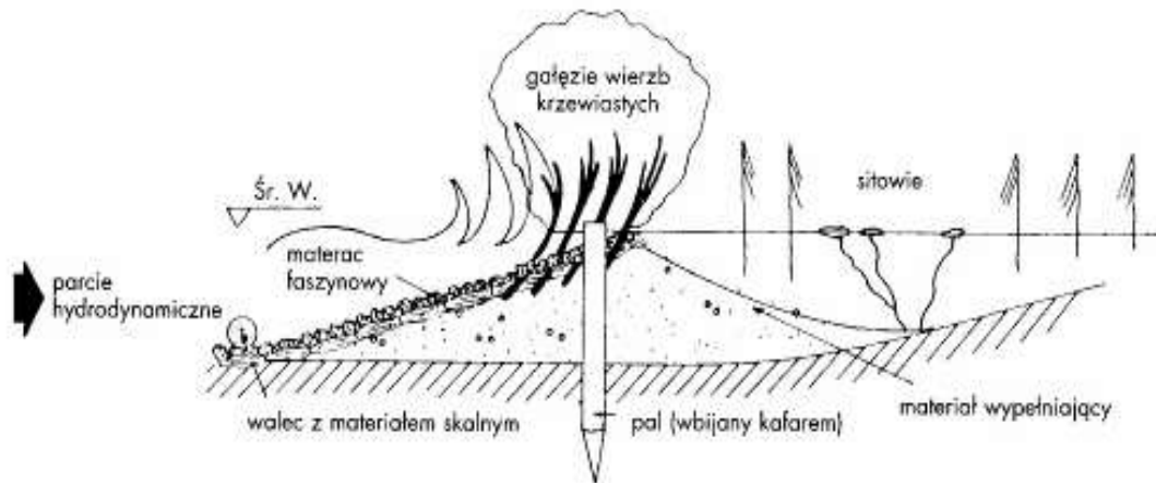
Tama faszynowa (Begemann i Schiechtl 1999)
