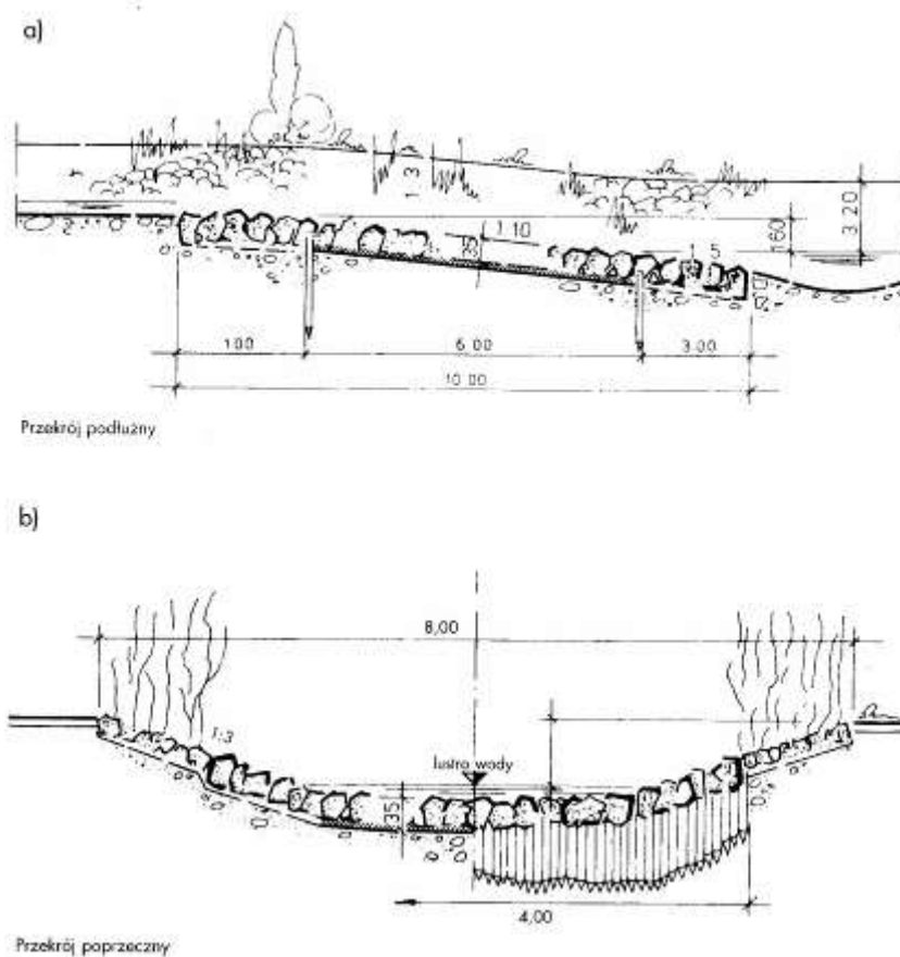
Bystrze z kamienia łamanego, stabilizujące dno (Begemann i Schiechtel 1999)
