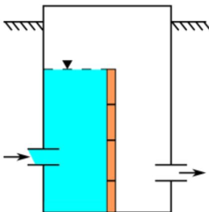
Studnia piętrząca na zbieraczu przed wylotem. Rys. P. Włodarczyk na podstawie Mioduszewski 2003.
