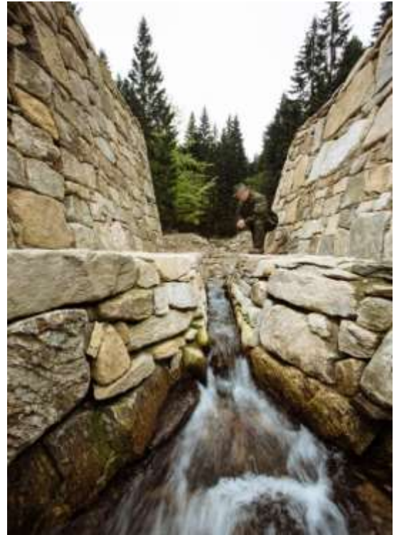
V-kształtny przelew wody ze zbiornika przeciwpowodziowego umożliwiający przejście rumowiska i samoczynne napełnianie i opróżnianie obiektu - Nadleśnictwo Międzyzlesie. Źródło: Archiwum CKPŚ. (rys. z prawej strony)
