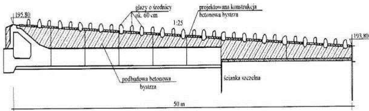
Rys. 8. Projekt przebudowy jazu stałego na przepławkę dla ryb (Mokwa i Wiśniewski 2008).
