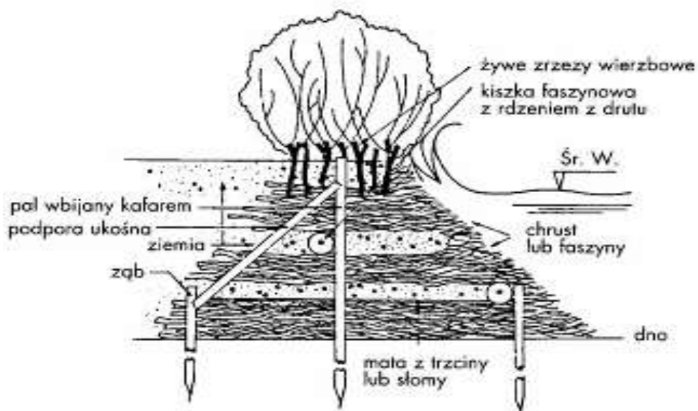
Żywa tama faszynowa (Begemann i Schiechtel 1999)
