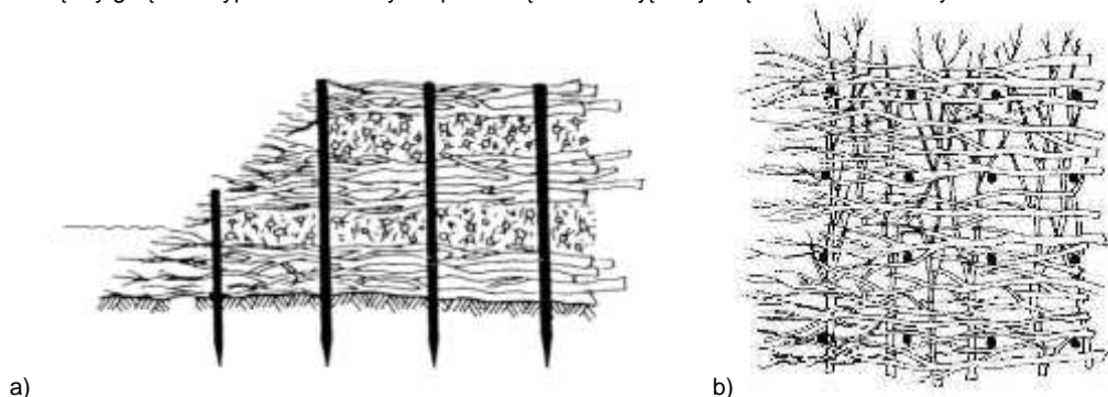
Brzegosłn krzyżowy a - przekrój poprzeczny, b – rzut z góry (Begemann i Schiechtl 1999)
