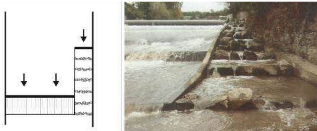
Przeplawka kaskadowa przy budowlu hydrotechnicznej. (Jelonek 2008)
