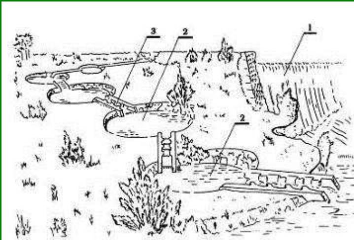
Przeplawka z połączonych akwenów (Żbikowski i Żelazo 1993, fot. M. Jelonek 2008): 1 – zapora/jaz 2 - akweny 3 - połączenia
