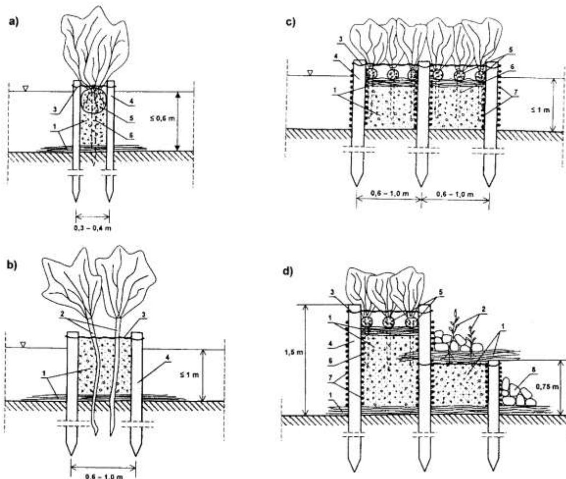
Konstrukcje faszynowo - palowe (Żelazo i Poppek 2002)
