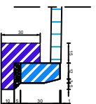
SZCZEGÓL KONSTRUKCYJNY
