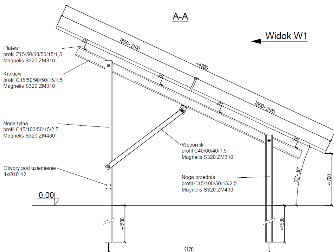
Rys.5. Przykładowa konstrukcja montażowa
