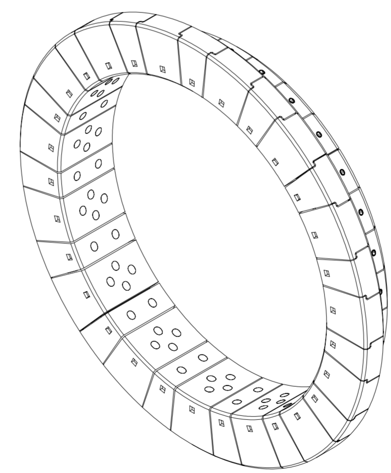
DÉTAIL E ECHELLE 1 : 10
