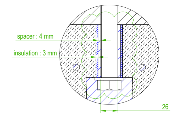
DÉTAIL D ECHELLE 1 : 3
