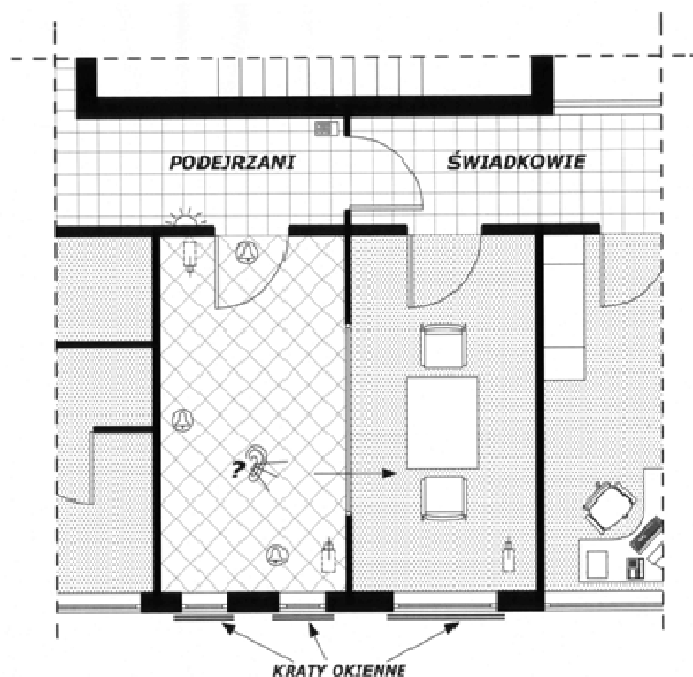
Rys. Przykład układu funkcjonalnego pokoju przesłuchań i okazań.
