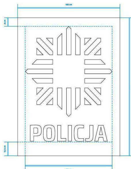
Rys. nr 1.10 Semafor – schemat wymiarowy
