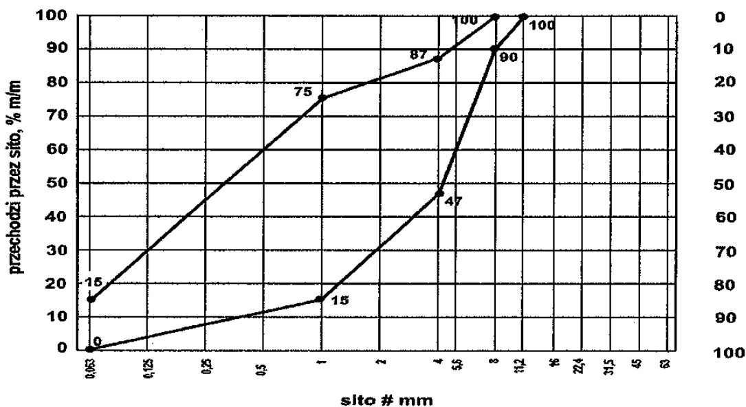
Rys 1. Mieszanka kruszyw 0/8 do górnej warstwy podłoża ulepszonego
