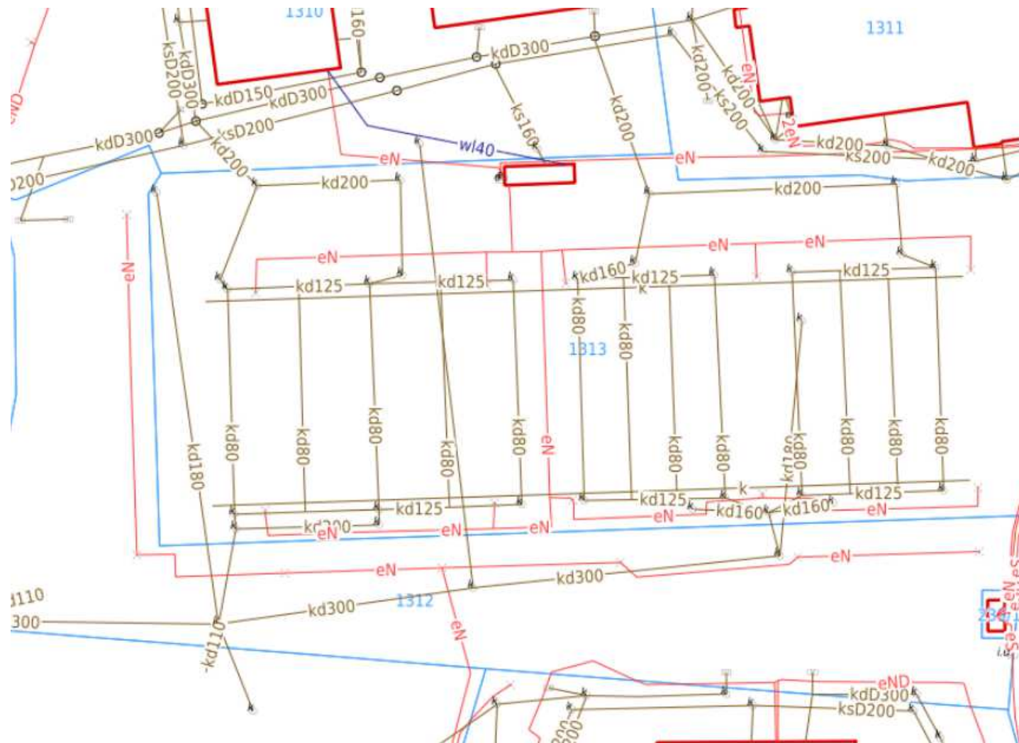
Rysunek 3 Istniejące uzbrojenie terenu
