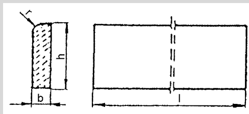
Rysunek 1. Kształt betonowego obrzeża Tablica 1. Wymiary obrzeży
