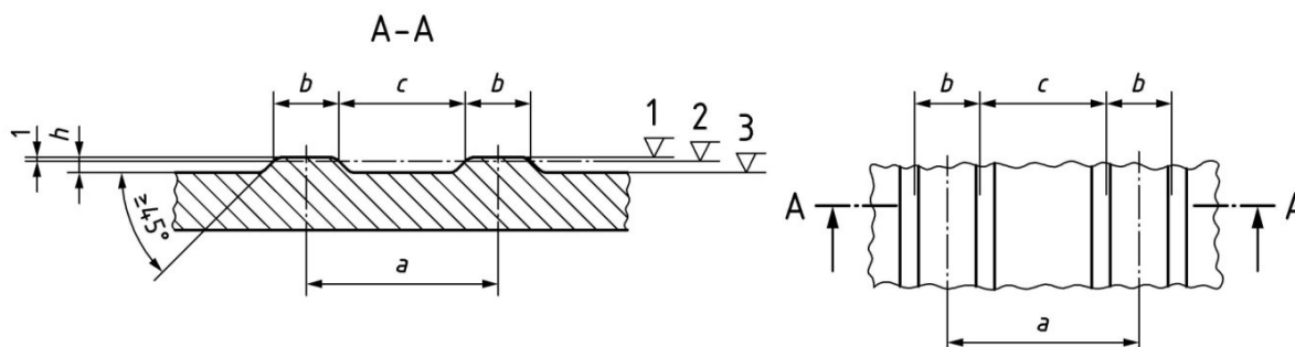
Rys. 1a. Płytki kierunkowe asymetryczna – prowadząca – szczegół powierzchni
