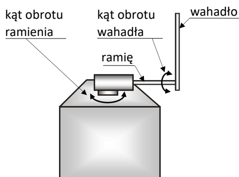
Rys. 1. Schemat poglądowy obrotowego wahadła odwróconego
