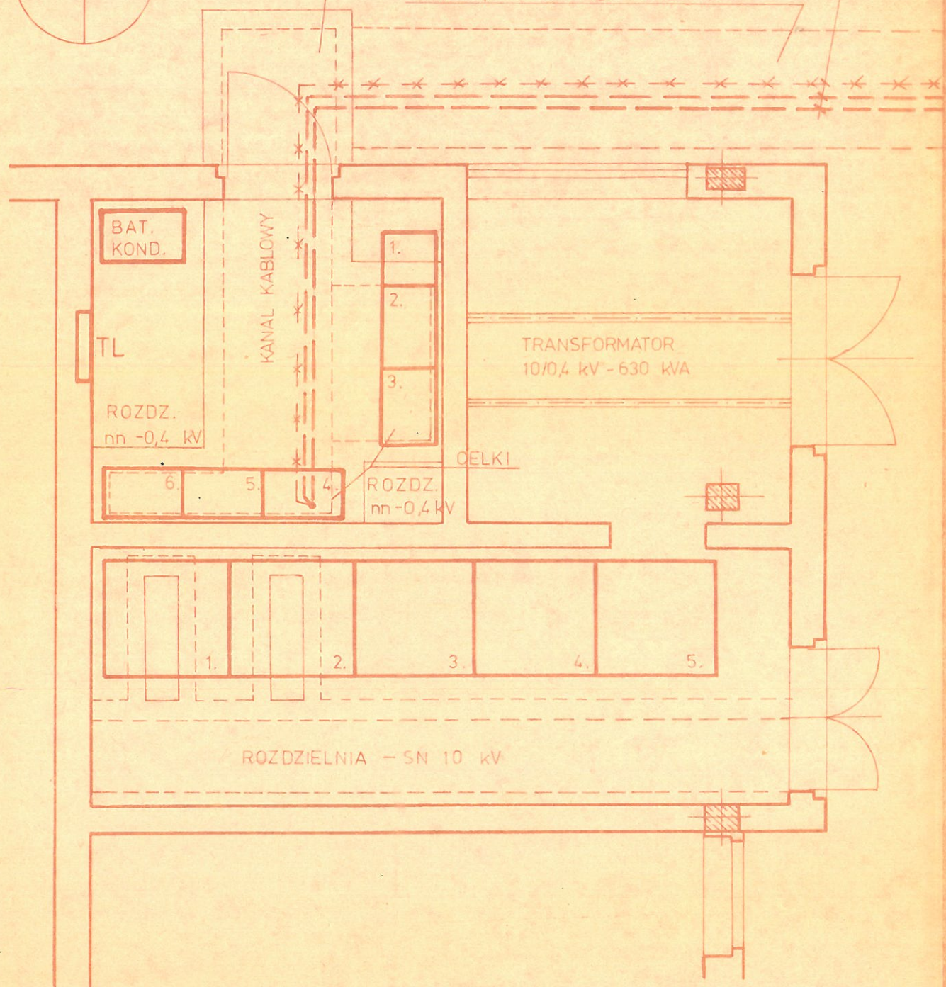
- RZUT PRZYZIEMIA -
