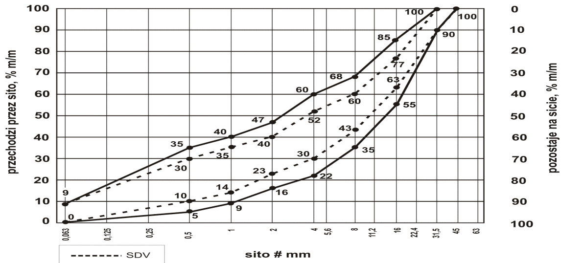
Rysunek 1. Mieszanka niezwiązana 0/31,5 do warstwy podbudowy pomocniczej z mieszanki niezwiązanej z kruszywem C90/3
