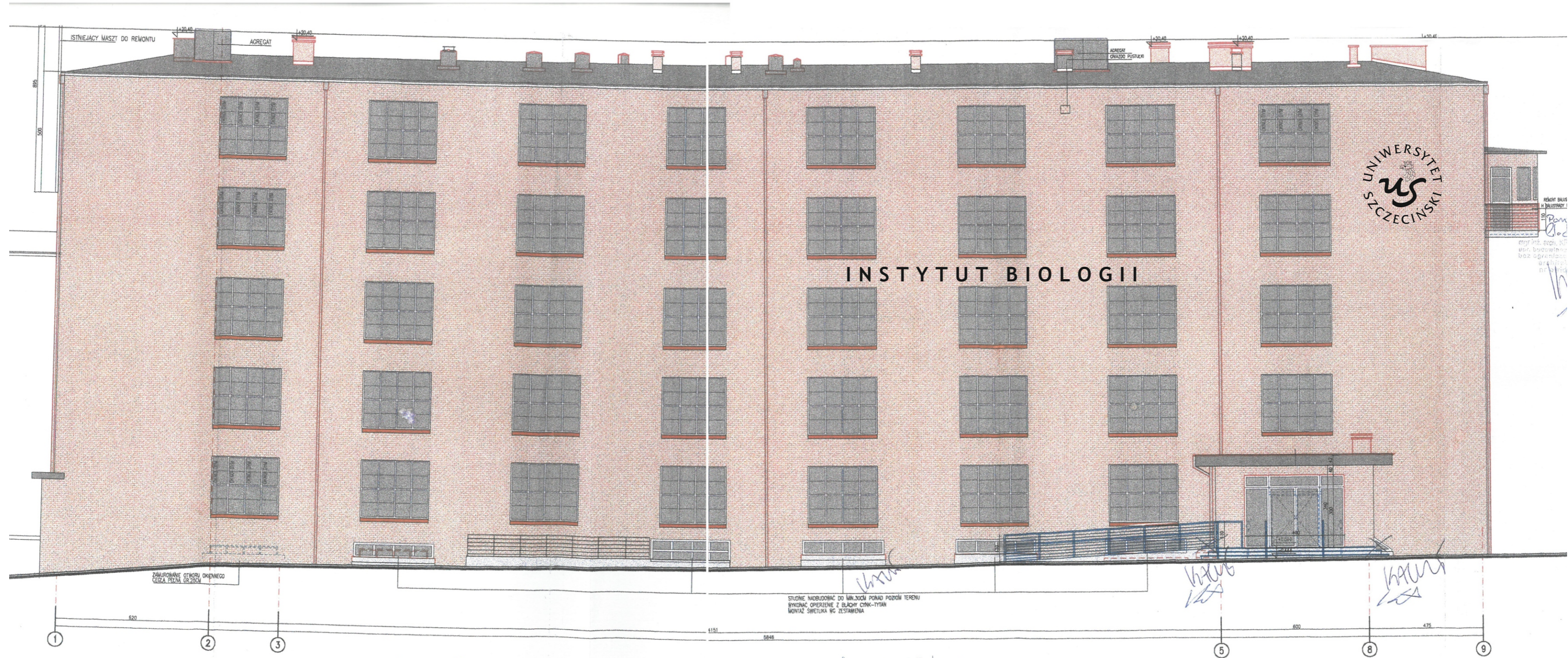
ELEWACJA ZACHODNIA
