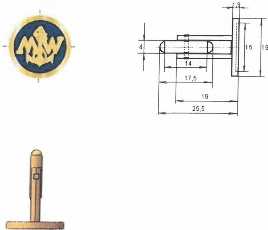
Rys. nr 4. Spinka marynarki wojennej (do mankietów)
