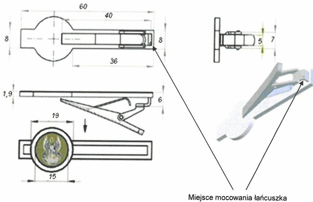
Rys. nr 5. Spinka wojsk lądowych (do krawata) Wzór 841D/MON
