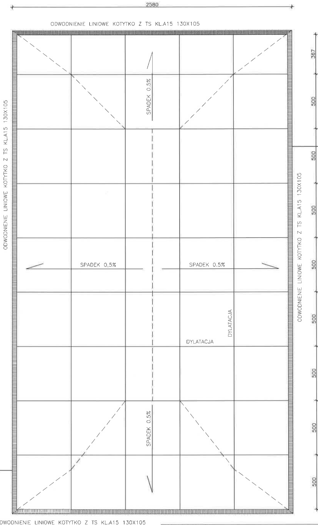
ODWODNIENIE LINIOWE KOTYTKO Z TS KLA.15 130X105
