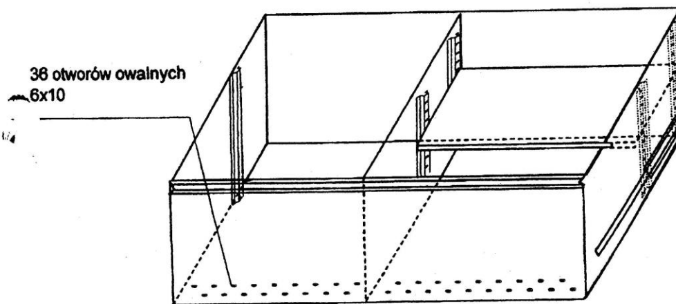
Szczegół F szuflada wysuwana
