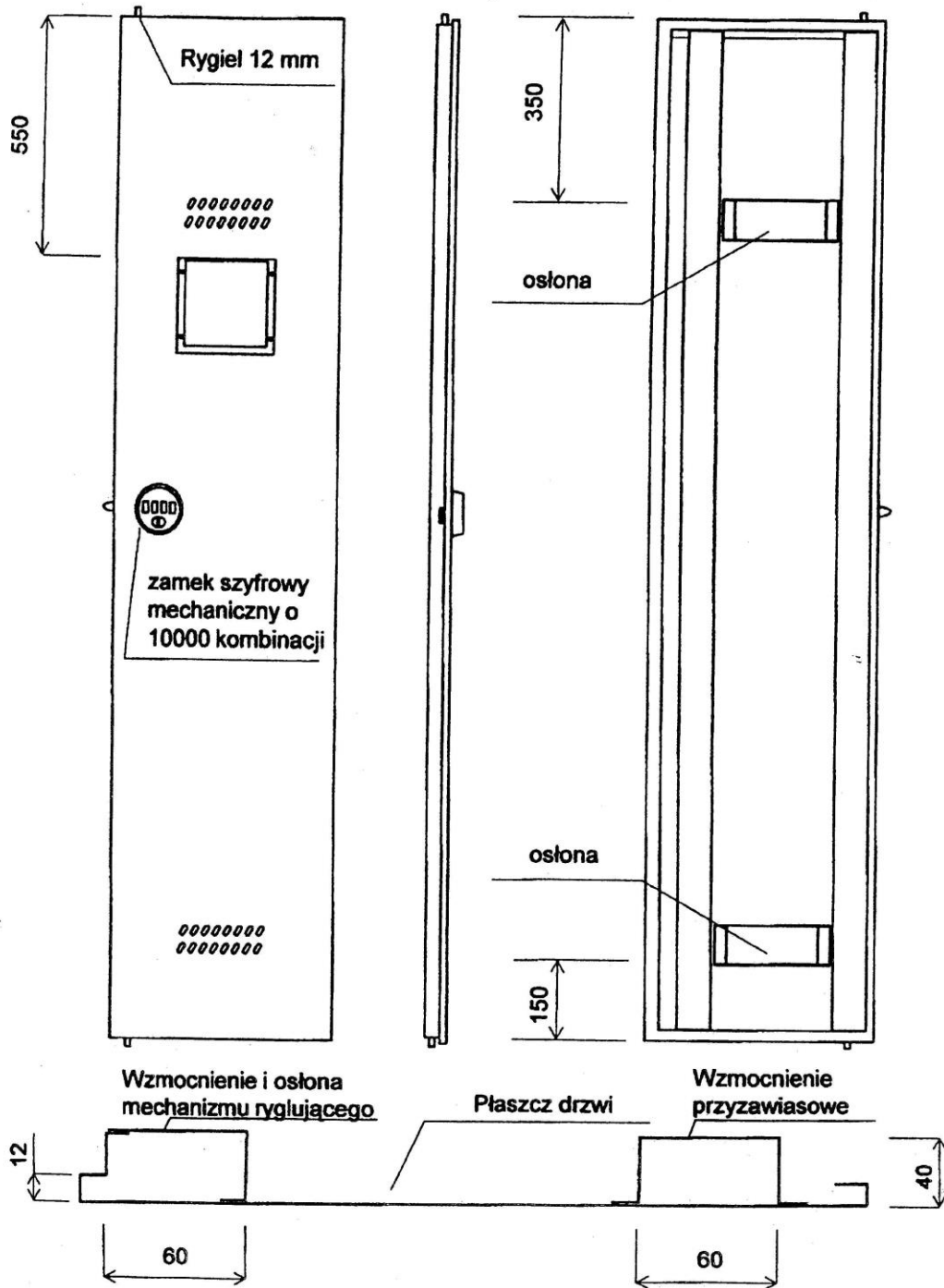
Szczegół J Drzwi prawe Rys. 9
