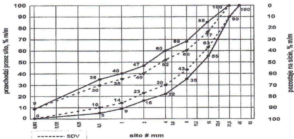
Rysunek 1. Mieszanka kruszyw 0/31,5 do warstw podbudowy zasadniczej
