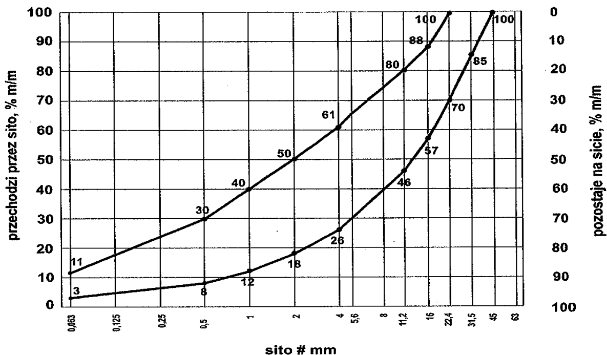
Rys. 1.1. Uziarnienie mieszanki CBGM 0/31,5
