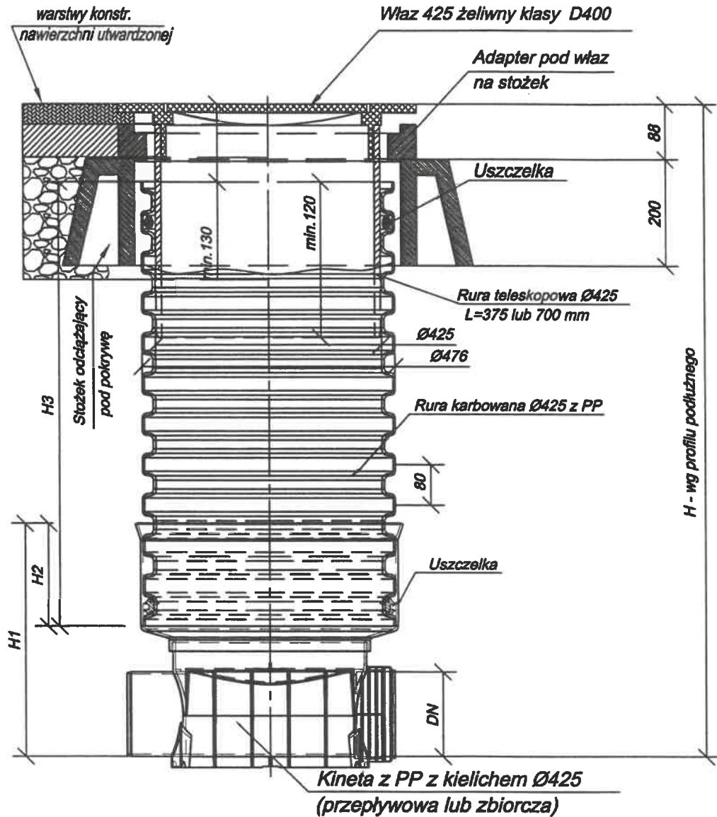
Studzienka inspekcyjna Ø425 z rurą trzonową karbowaną DN425 (z rurą teleskopową i włazem żeliwnym D400 na stożku odciążającym) z kinetą przepływową lub zbiorczą
