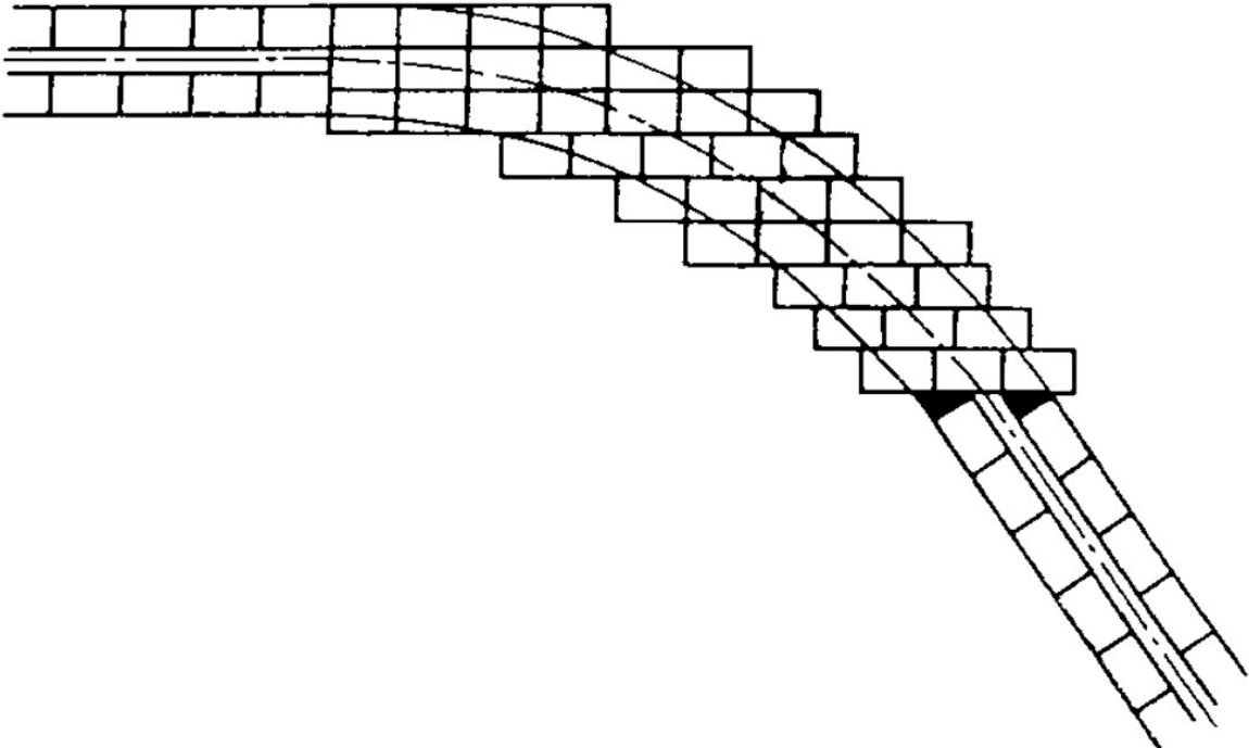
Rys. 5. Układanie płyt na łuku o małym promieniu
