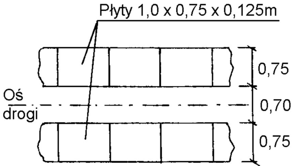
Rys. 2. Przykłady ułożenia płyt na jezdni jednopasowej System pasowy – wariant 1
