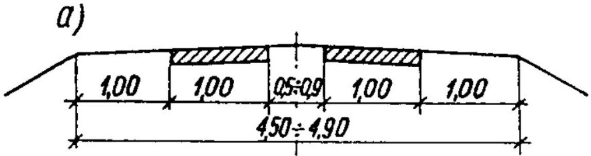
Rys. 4. Przekroje poprzeczne dróg z nawierzchniami z płyt, ułożonymi w systemie pasowym
