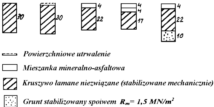
Rys. 4. Przyk6adowe wybrane konstrukcje nawierzchni utwardzonego pobocza z kruszywa łamanego niezwi6zanego
