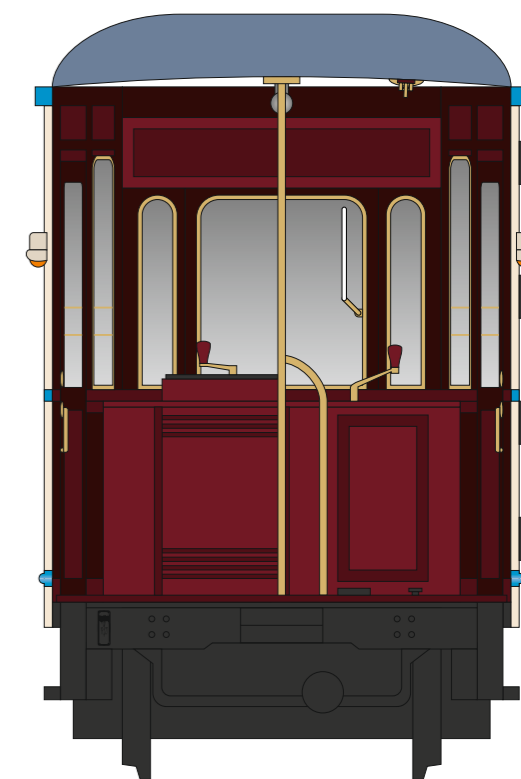
Rys. 2.2. Widok przekrojowy frontowy B-B'
