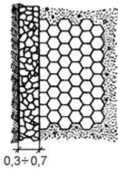
Rys. 2. Widok z góry obramowania z brukowca przy jezdni z płyt betonowych sześciokątnych (trylinki)
