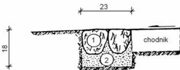
Rys. 4. Obramowanie chodnika z brukowca wysokości 10÷12 cm
