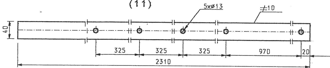
Cięgno przesypu 1:5 (11)
