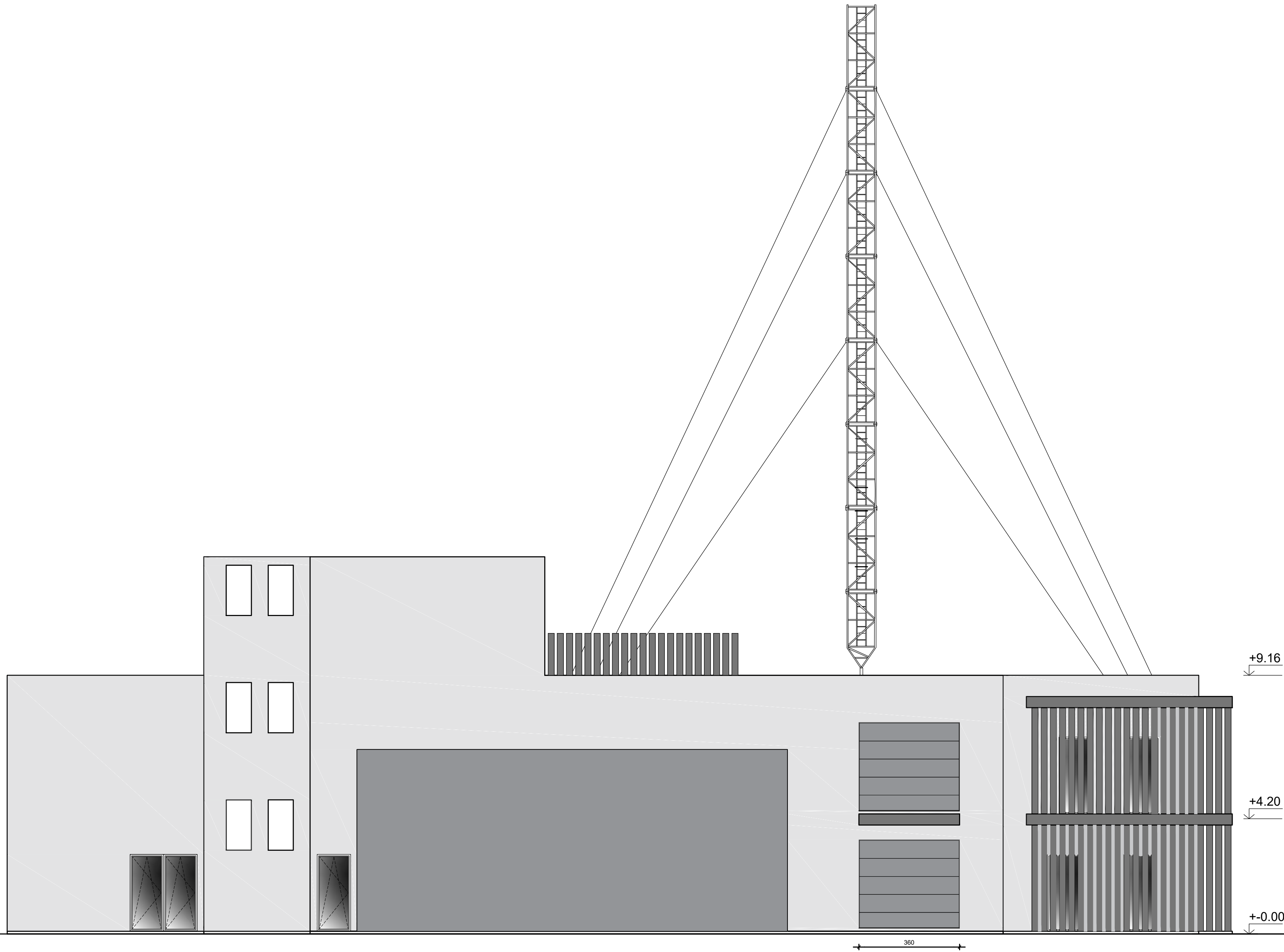
ELEWACJA PÓŁNOCNA
