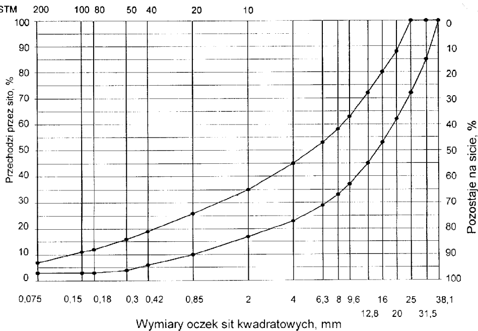
Rys.1. Krzywe graniczne uziarnienia mieszanki mineralnej BA od 0 do 31,5 mm do podbudowy nawierzchni drogi o obciążeniu ruchem KR 1 lub KR 2
