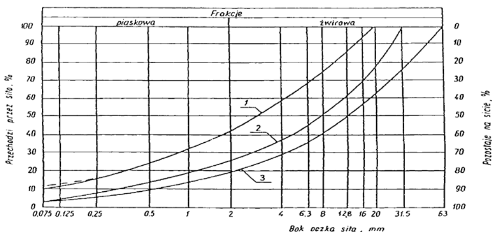
Rysunek 1. Pole dobrego uziarnienia kruszyw przeznaczonych na warstwy ulepszonego podłoża i podbudowy wykonywanych metodą stabilizacji mechanicznej
