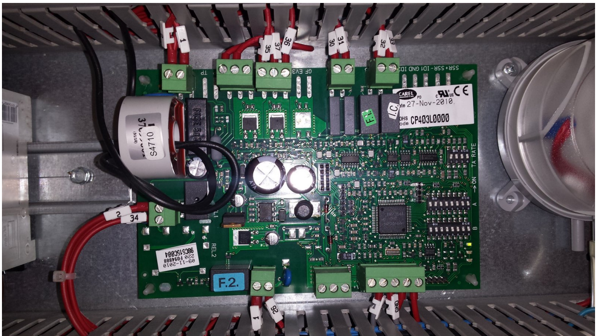
Sterownik nawilżacza.
