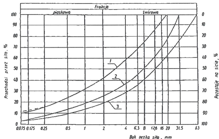
1-2 kruszywo na podbudowę zasadniczą (górną warstwę) lub podbudowę jednowarstwową, 1-3 kruszywo na podbudowę pomocniczą (dolną warstwę)
